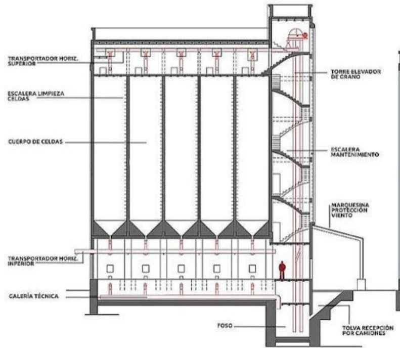
1946_Seccion de silo de grano_Red Nacional de Silos
