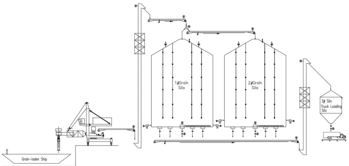
2002_Diagrama de Funcionamiento de Silo Portuario
