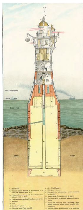
1908_Faro de Weser_Seccion Ilustrativa
